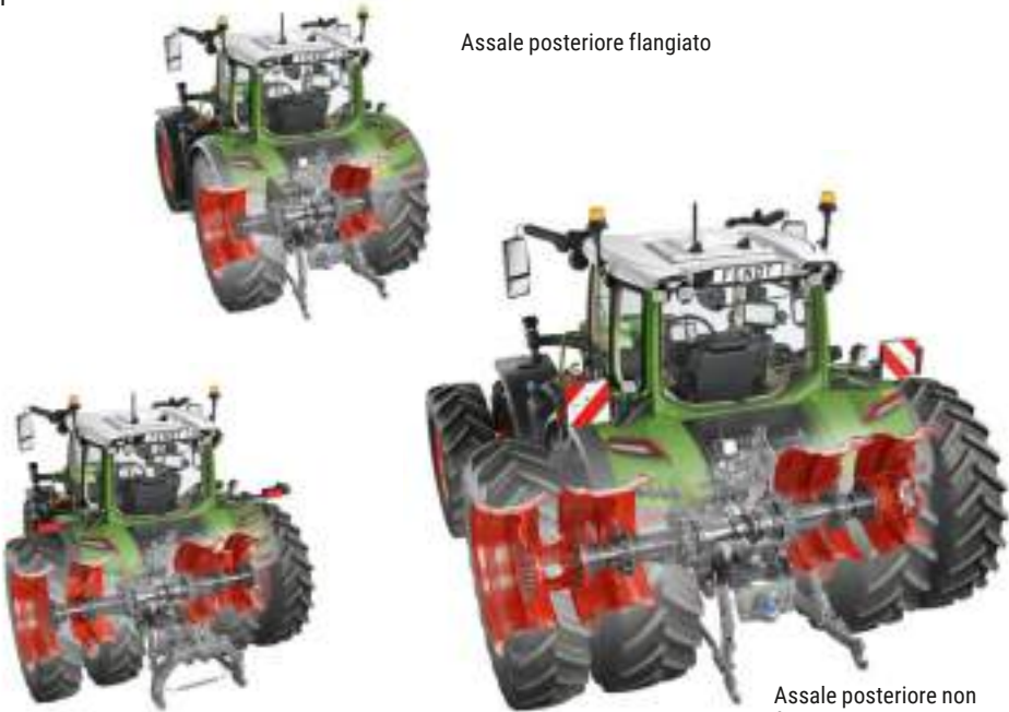
Assale posteriore non flangiato 2500 mm con pneumatici gemellati e mozzo doppio
